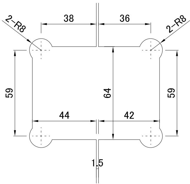
182.elt ガラス加工図
