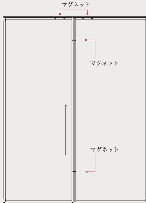
マグネット取り付け No2 二重回転式ガラスドア、均等パネル ■DFRマグホルド 左 or 右
