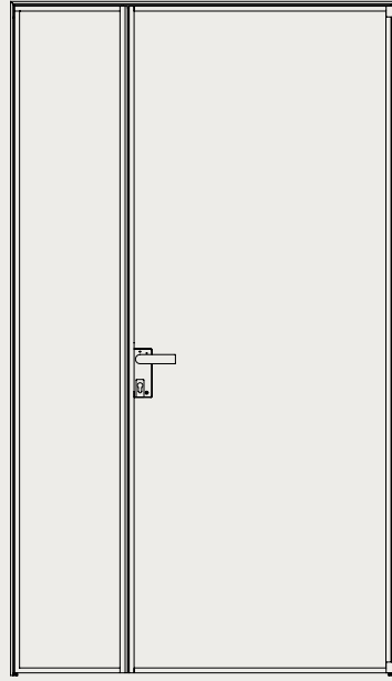
ロックアプリケーション No2 サイド固定ドアパネル付きシン グルピボットガラスドア ■DFR MECロック ■DFRマグネットロック 左 or 右
