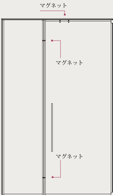
マグネット取り付け No4 固定パネル付きシングルピボットガラスドア ■DFRマグネットホルド 左 or 右
