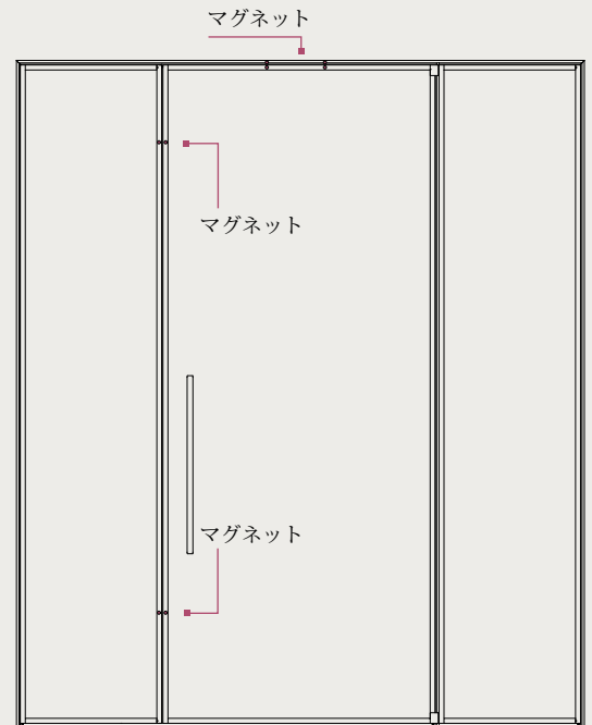
マグネット取り付け No3 固定パネル付きシングルピボットガラスドア ■DFRマガジンホルド 左 or 右
