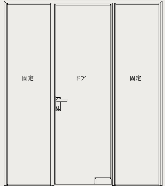
ノスカボアプリケーション No3 固定パネル2枚付きシングルピボットガラスドア DFR ノスカボ ■DFR MECロック ■DFR マグネットロック 左 or 右
