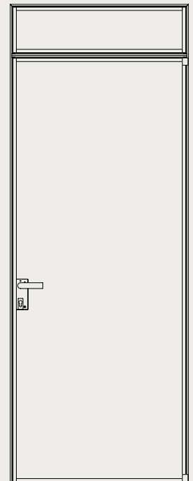
ロックアプリケーション No6 上部固定パネル付きシングル ピボットガラスドア固定パネル ■DFR MECロック ■DFR マグネットロック ■DFR マグネットホルド 左 or 右
