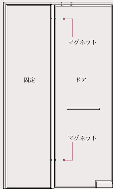
ノスカボアプリケーション No6 固定パネル付きシングルピボットガラスドア、 DFR ノスカボ ■DFR マグホールド 左 or 右
