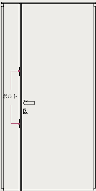
ロックアプリケーション No4 ボルト付きサイド可動ドアパネル付き ダブルピボットガラスドア ■DFR MECロック ■DFRマグネットロック ■ボルトロック 左 or 右
