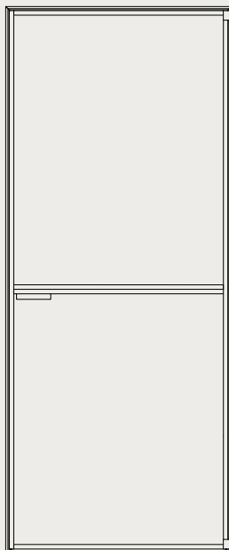
分割アプリケーション No1 ガラス仕切り付き シングルピボットガラスドア ■マグホールド 左or右
