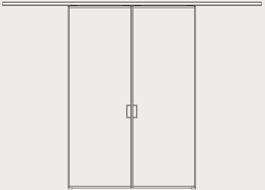
スライド式ドア用アプリケーション No2 両開きスライド式ガラスドア ■ドアハンドル ■スライド式ロック
