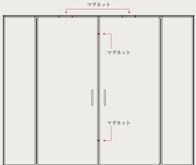
マグネット取り付け No5 固定パネル2枚付きダブルドア ■DFRマグネットホルド 左 or 右
